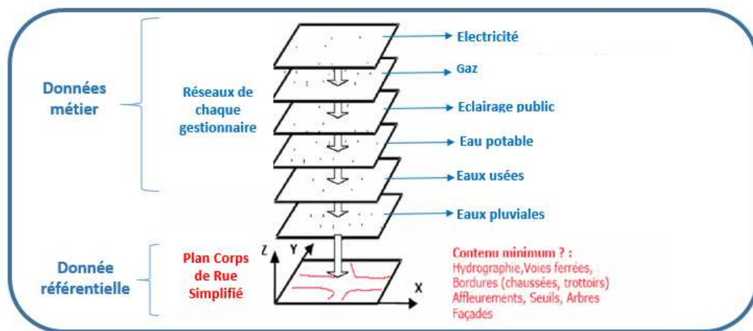
Fig. n°1 : Le PCRS : la couche de base de tous les réseaux
